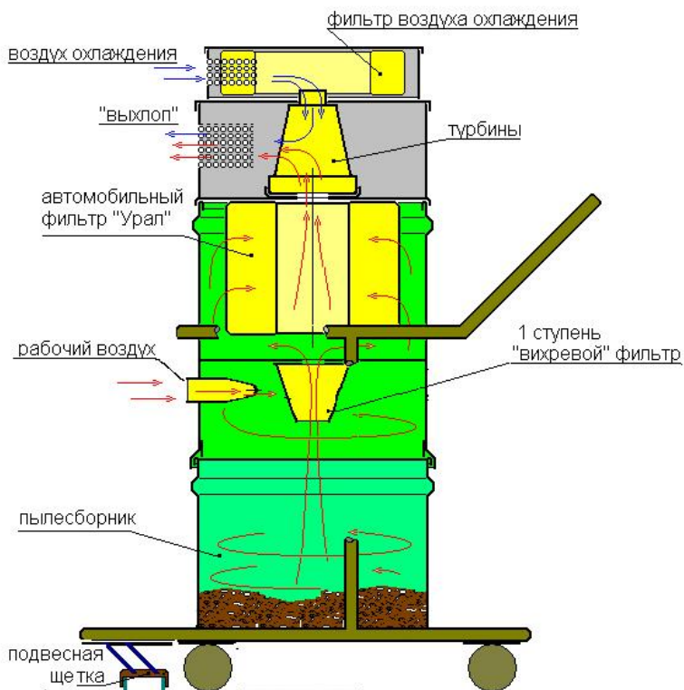
Рис. 1. Схема пылесоса
