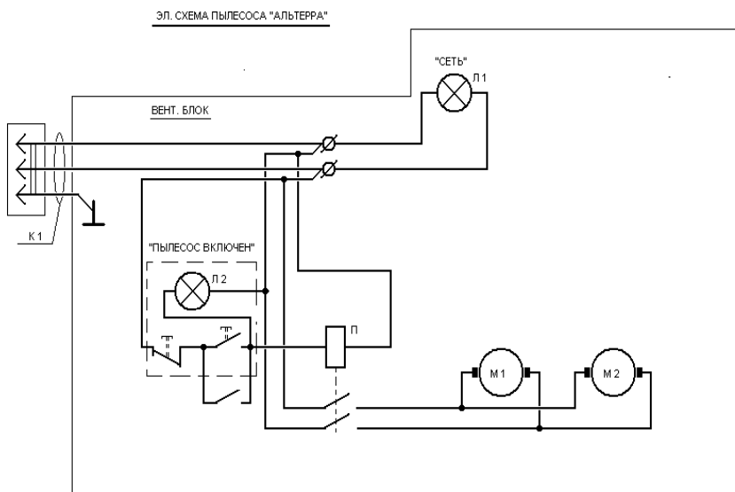
Рис. 3. Схема электрическая принципиальная
